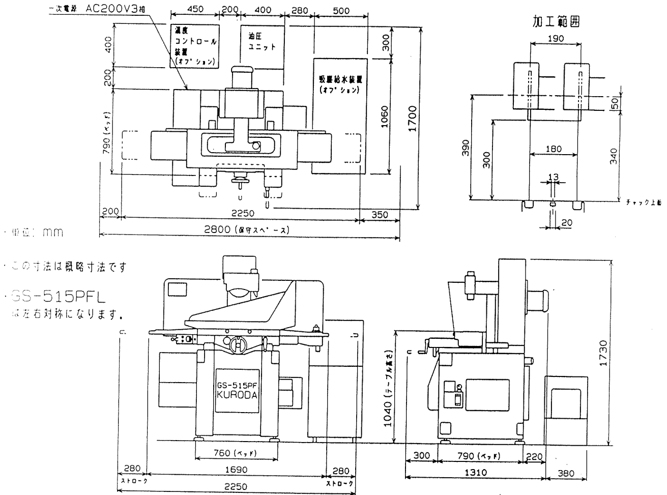
図 1-3 機械の寸法
